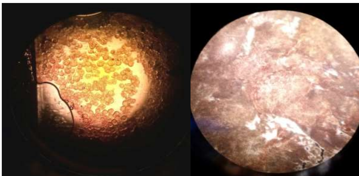
شکل ۳: بافت اندام‌های جنسی نر (سمت راست) و ماده (سمت چپ) کپور معمولی در سن هفت ماهگی تهیه‌شده با روش استوک‌کارمن. Figure 3: gonad histology of female (left) and male (right) common carp using Aceto-Carmine squash method in the age of seven months.
