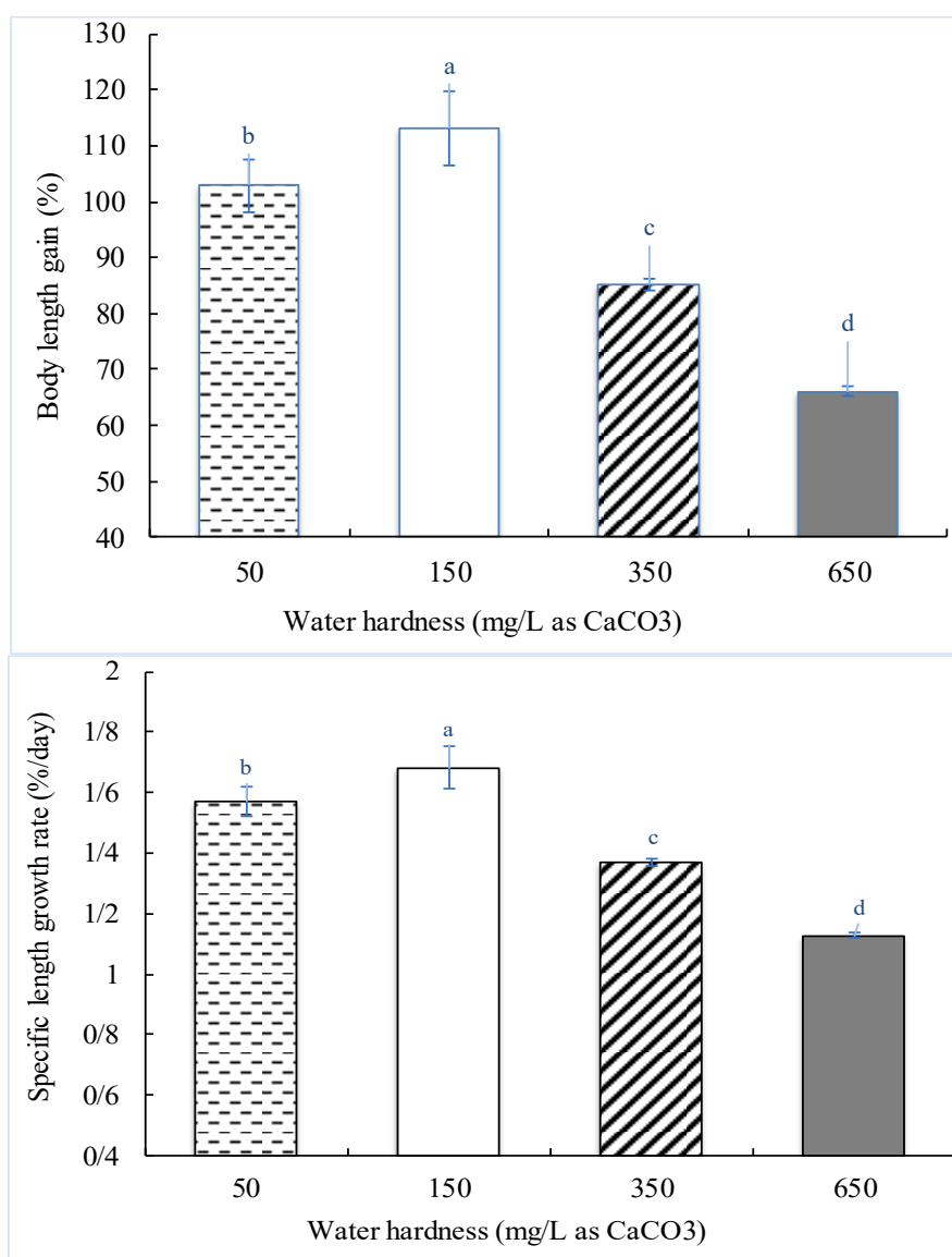
شکل ۲: درصد افزایش طول بدن و نرخ رشد ویژه طولی (درصد در روز) در گربه‌ماهی خال‌طلایی ( Pterygoplichthys joselimaianus ) پرورش یافته در سطوح مختلف سختی آب (میلی‌گرم بر لیتر کربنات کلسیم)
