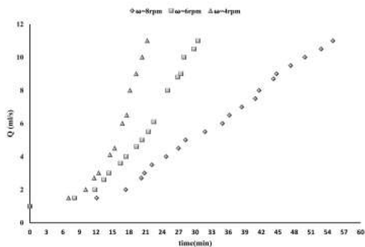
شکل ۳ الف: نمودار افت-زمان برای دبی ورودی ۵۵۰ میلی‌لیتر بر ثانیه (سطح غرقابی ۱۵ درصد و غلظت ۳۰ میلی‌گرم بر لیتر) در سرعت‌های چرخشی ۸ دور بر دقیقه ( SEM^4 = ۰/۰۵۱ )، ۶ دور بر دقیقه ( SEM = ۰/۰۰۶ ) و ۴ دور بر دقیقه ( SEM = ۰/۰۵۸ ).
