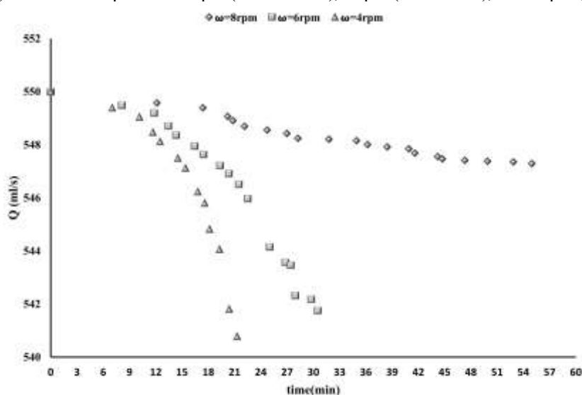
شکل ۳ ب: نمودار دبی-زمان برای دبی ورودی ۵۵۰ میلی‌لیتر بر ثانیه (سطح غرقابی ۱۵ درصد و غلظت ۳۰ میلی‌گرم بر لیتر) در سرعت‌های چرخشی ۸ دور بر دقیقه ( SEM = ۰/۰۵۱ )، ۶ دور بر دقیقه ( SEM = ۰/۰۰۶ ) و ۴ دور بر دقیقه ( SEM = ۰/۰۵۸ ).
