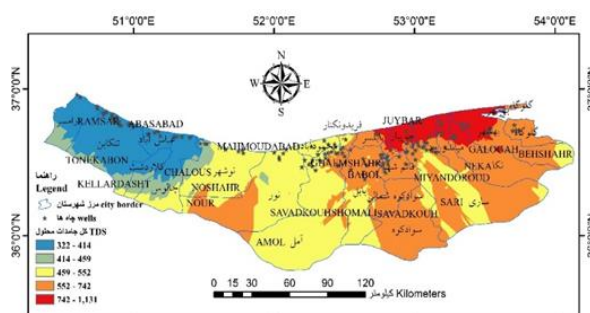
شکل ۶: وضعیت جامدات محلول آب چاه‌ها در محدوده‌ی مطالعاتی
