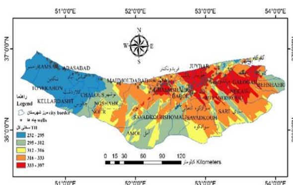
شکل ۷: وضعیت سختی کل آب چاه‌ها در محدوده‌ی مطالعاتی
