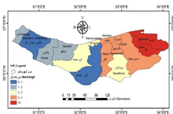
شکل ۸: وضعیت دبی مصرفی برحسب لیتر بر ثانیه برای تولید هر تن ماهی در محدوده‌ی مطالعاتی
