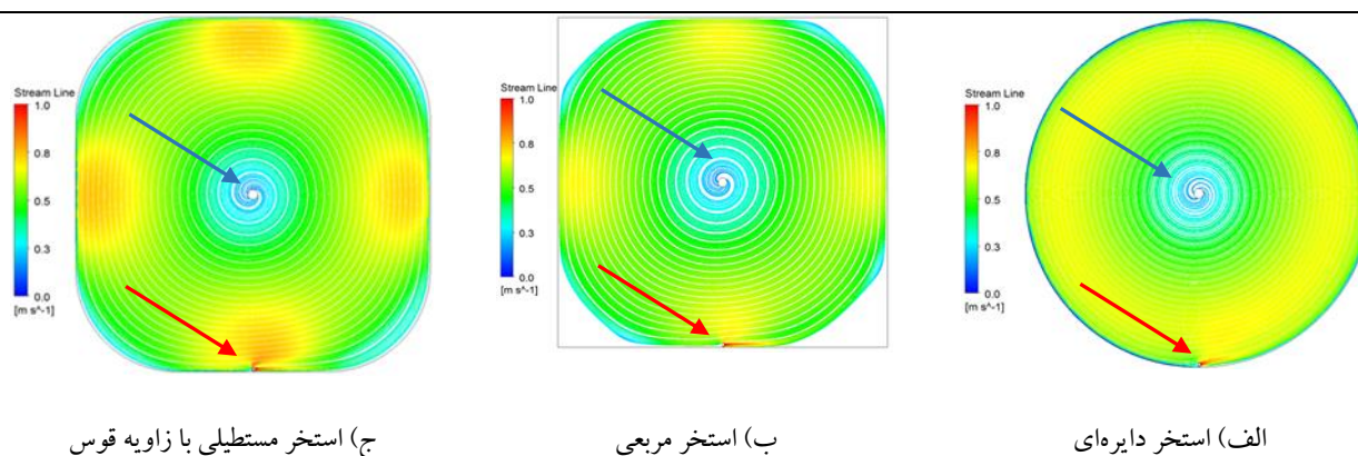
شکل ۳. مقایسه خطوط جریان برای پیکربندی های هندسی استخرهای مطالعاتی. پیکان قرمز نشان دهنده مکان ورودی بوده و پیکان آبی مکان خروجی را نشان می دهد.
