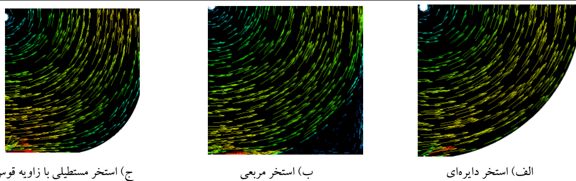
شکل ۵: بزرگنمایی مقایسه بردارهای سرعت در گوشه‌های استخرهای مطالعاتی که نشان‌دهنده نمای از نزدیک چرخه‌های ایجاد شده در مجاورت گوشه‌های استخرهای مطالعاتی.
