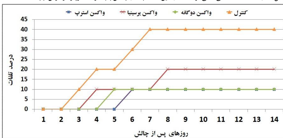
شکل ۵: درصد تلفات تجمعی ماهی قزل آلائی رنگین کمان بعد از چالش با باکتری یرسینیا راگری
