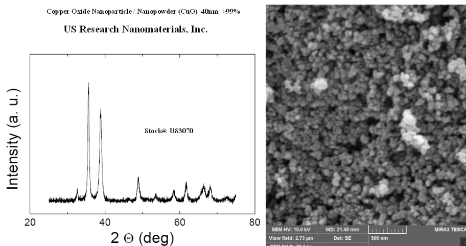
شکل ۱: تصویر الکترونی نگاره (SEM) Scanning Electron Microscopy و نمودار طیف پراش اشعه X (X-ray) نانوذرات اکسید مس
