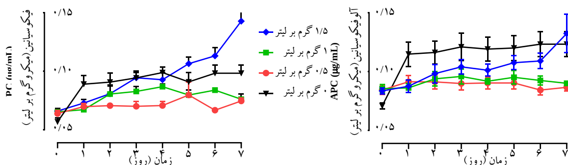
شکل ۷: تغییر محتوای رنگدانه فیکوسیانیین و آلفوفیکوسیانیین با غلظت در محیط کشت حاوی منبع کربنی جایگزین
