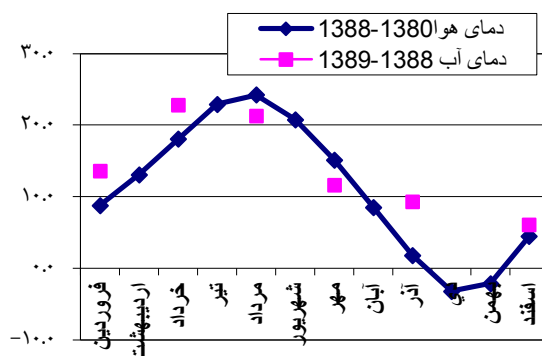
شکل ۵: میانگین دمای آب و هوا در سد گلابره زنجان
