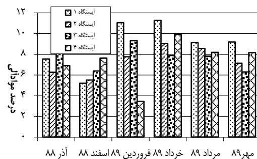
شکل ۴: میانگین درصد مواد آلی در رسد مخزنی گلابره
