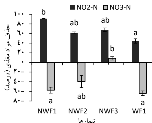
شکل ۴: درصد میزان حذف فاکتورهای نیتريت (NO 2 -N) و نترات (NO 3 -N) در تیمارهای مختلف طی دوره آزمایش (حروف انگلیسی غیر مشترک نشان دهنده تفاوت معنی دار میانگین تیمارها با یکدیگر می باشند)
