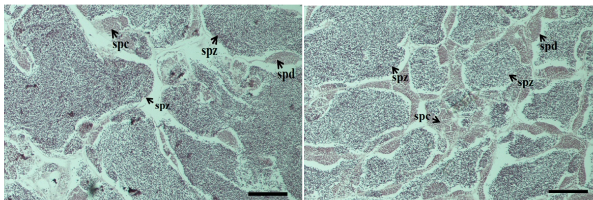
شکل ۱: بافت گناد نر ماهی سفید دریای خزر ساکن رودخانه قشلاق سندج با بزرگ‌نمایی \times 400 : spc: اسپرماتوسیت، spd: اسپرماتید. Spz: اسپرماتوزآ. (۱۰۰ میکرومتر). Spz: اسپرماتوزآ.
