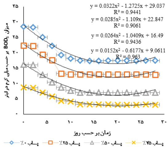
شکل ۶ ب: تغییرات BOD 5 در تیمارهای به کار رفته در این آزمایش طی ۲۸ روز
