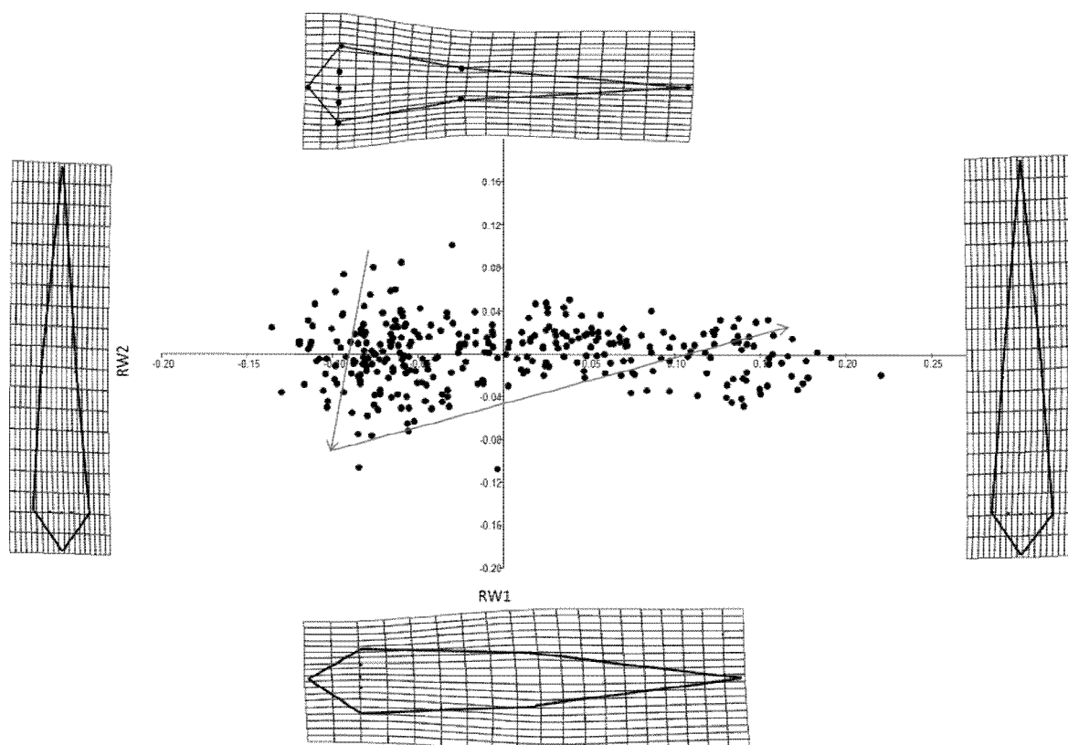
شکل ۲: پراکندگی داده‌های مربوط به آنالیز Relative warp نمونه‌های ماهی صبیتی S. hasta از روز اول بعد از تفریخ تا ۳۵ روز بعد از آن در طول محور RW1 و RW2. نمونه‌های کم سن‌تر از شماره ۱ و نمونه‌های با سن بیشتر با اعداد بزرگتر علامت‌گذاری شده‌اند.
