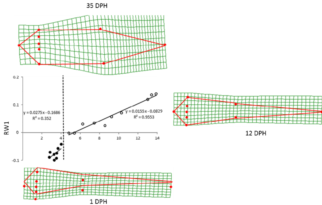
شکل ۳: روند رشد ماهی صیبتی S. hasta از روز اول پس از تفریخ تا ۳۵ روز بعد از آن براساس پراکندگی داده‌های مربوط به RW1 نسبت به طول کل (خط چین نشان‌دهنده نقطه عطف است).
