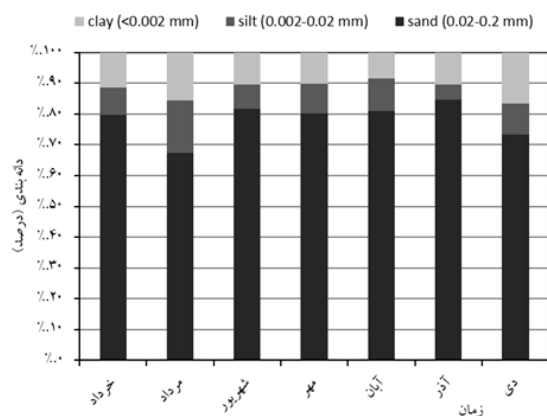
نمودار ۸: میزان دانه‌بندی رسوبات شنی اندازه‌گیری شده در داخل قفس
