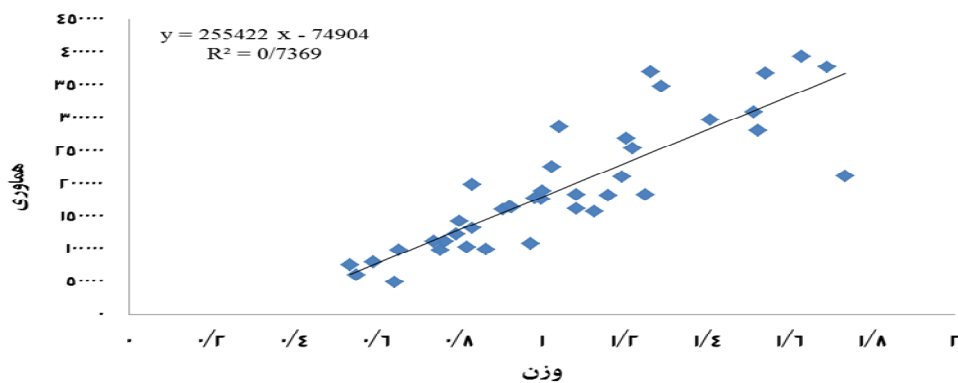
شکل ۳: رابطه میزان هماوری مطلق با وزن در کرم پرتار P. nuntia در سواحل بندرعباس
