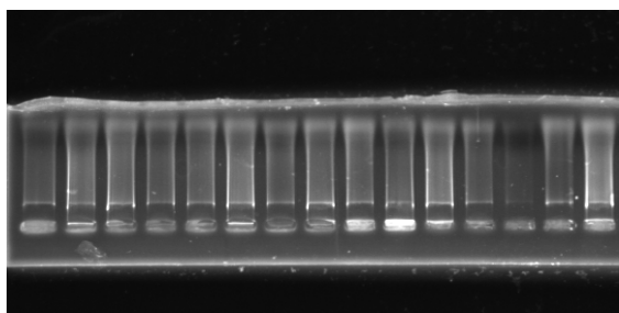
شکل ۲: ارزیابی DNA استخراج شده شبه شوریده در نواحی مورد بررسی به روش اسنات آمونیم
