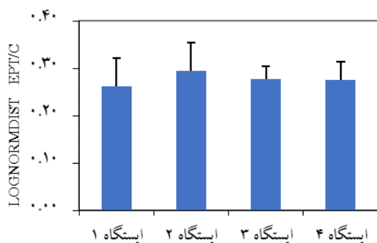
شکل ۱۶. مقدار میانگین نرمال شده لگاریتمی شاخص EPT/C
