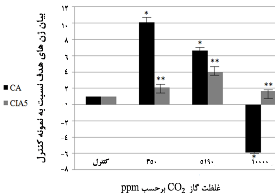
شکل ۲. مقایسه تغییرات وابسته به گاز CO 2 در میزان mRNAهای مربوط به دو ژن CAB و CIA5 . سطوح رونوشت به عنوان مقدار نسبی رونوشت‌های ارجاع شده به بیان ژن نمونه رشد یافته در غلظت ۱۰۰ ppm از گاز CO 2 گزارش شده است.
