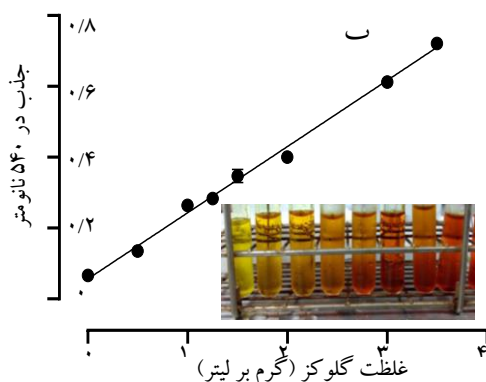
شکل ۲: الف) نمودار اعتبارسنجی طول موج، ب) نمودار استاندارد تعیین قند احیاکننده به روش DNS (داده‌های نمودارها میانگین ۳ تکرار را نشان می‌دهد).
