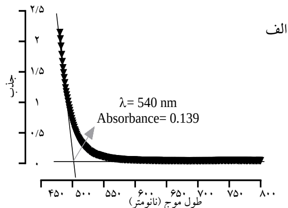
شکل ۲: الف) نمودار اعتبارسنجی طول موج، ب) نمودار استاندارد تعیین قند احیاکننده به روش DNS (داده‌های نمودارها میانگین ۳ تکرار را نشان می‌دهد).
