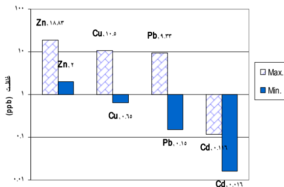
شکل ۲: مقادیر حداقل و حداکثر فلزات در آب کارگاه تکثیر و پرورش ماهیان خاویاری شهید دکتر بهشتی
