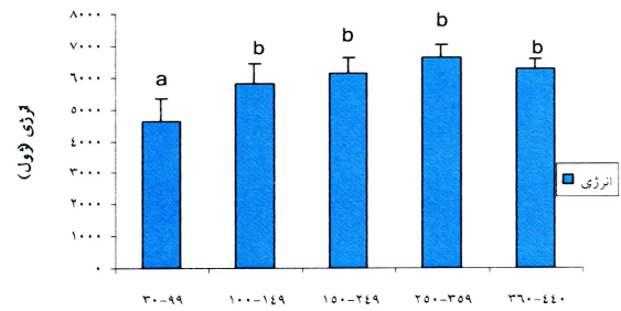
شکل ۴: میزان نترژی ترکیبات بدن در محدوده طولی متفاوت در ماهی بنی
