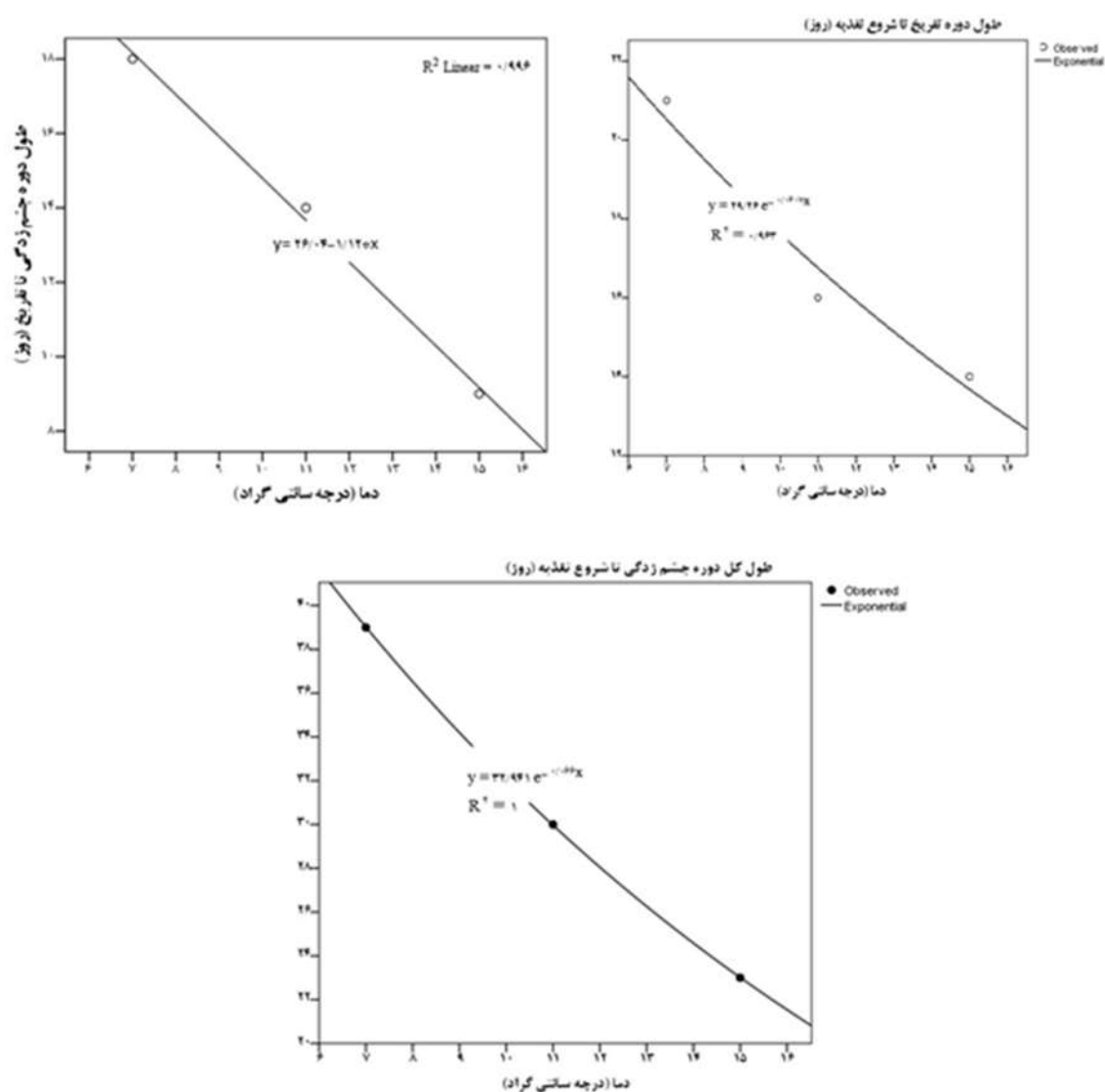
شکل ۱: تأثیر دما بر مدت زمان تکامل از تخم چشم زده تا تفریخ، تفریخ تا شروع تغذیه و کل دوره چشم زدگی تا شروع تغذیه (روز) در ماهی قزل آلا رنگین کمان
