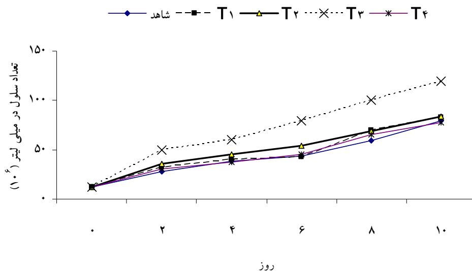
شکل ۲: تراکم (تعداد سلول در میلی لیتر \times 10^6 ) میکرو جلبک کلرلا در غلظت‌های مختلف پی کربنات سدیم
