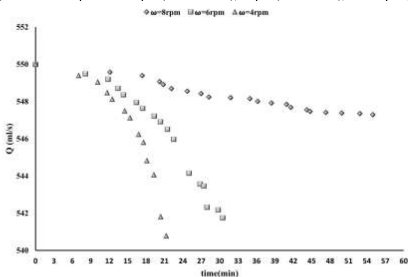
شکل ۳ ب: نمودار دبی-زمان برای دبی ورودی ۵۵۰ میلی‌لیتر بر ثانیه (سطح غرقابی ۱۵ درصد و غلظت ۳۰ میلی‌گرم بر لیتر) در سرعت‌های چرخشی ۸ دور بر دقیقه ( SEM=0.051 )، ۶ دور بر دقیقه ( SEM=0.06 ) و ۴ دور بر دقیقه ( SEM=0.058 ).
