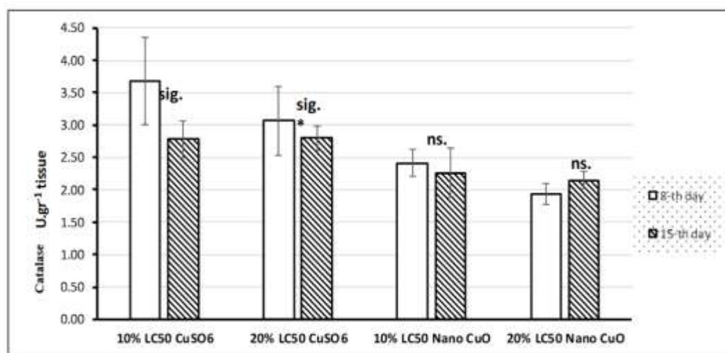
شکل ۳: مقدار کاتالاز در گاماروسهای در معرض دو ماده سولفات مس CuSO 4 و نانو اکسید مس Nano CuO بر اساس ۱۰ و ۲۰ درصد LC50 96h بعد از ۸ و ۱۵ روز
