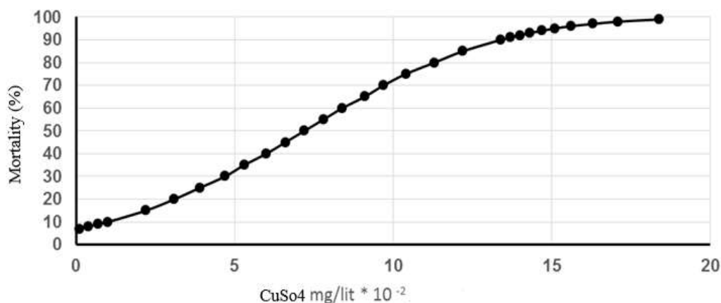
شکل ۱: نمودار برآورد تلفات گاماروس Gammarus pseudosyriacus در غلظت‌های مختلف سولفات مس
