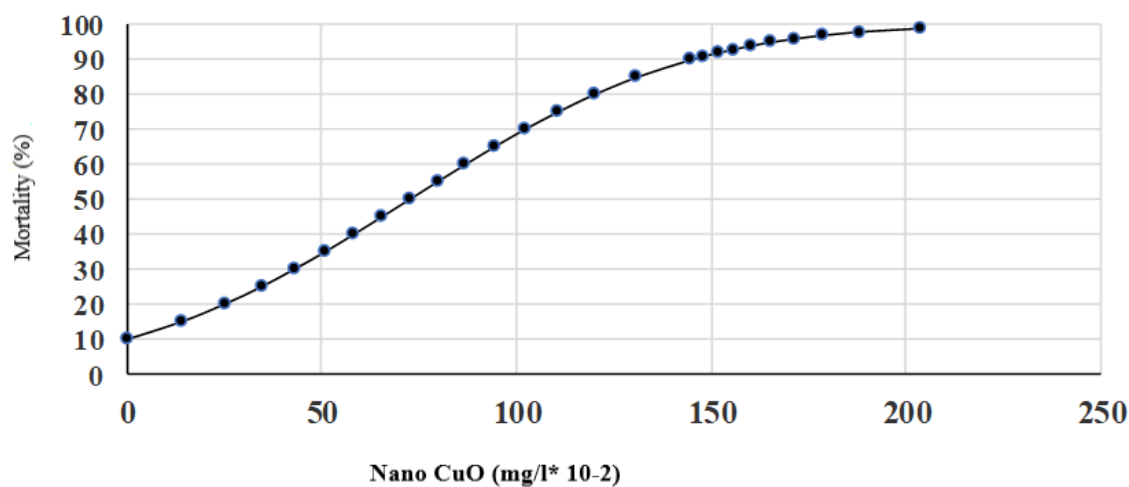
شکل ۲: نمودار برآورد تلفات گاماروس Gammarus pseudosyriacus در غلظت‌های مختلف نانو ذرات مس
